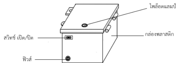
ภาพที่ 9 แบบร่าง 3 มิติ (มุมมองด้านข้างกล่อง)
