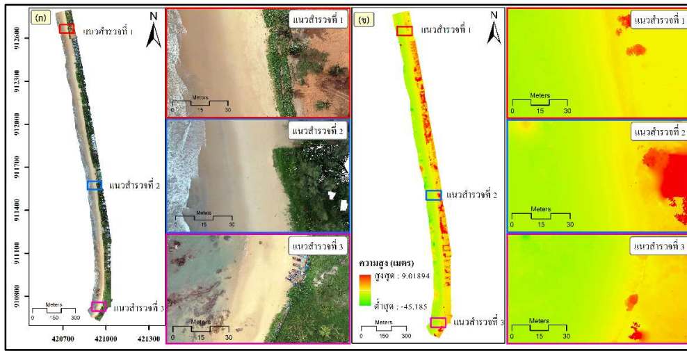
รูปที่ 5 ภาพออร์โธรีเฟอเรนซ์ (ก) แบบจำลองความสูงพื้นผิวเชิงเลข (ข) ที่ได้จากการประมวลผลภาพถ่ายจาก UAV
