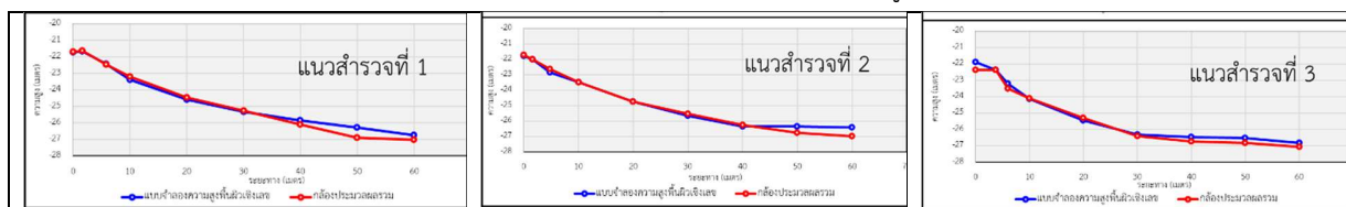
รูปที่ 7 ความสอดคล้องของภาพตัดขวางชายหาดจากการสำรวจจริงและแบบจำลองความสูงพื้นผิวภูมิประเทศ
