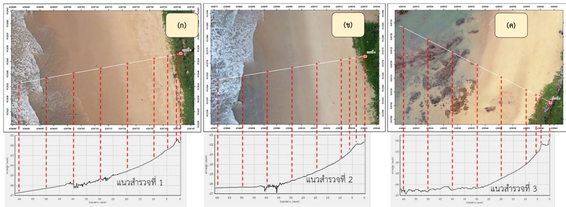
รูปที่ 6 ลักษณะฐานทรายหาด แนวสำรวจที่ 1 (ก) แนวสำรวจที่ 2 (ข) แนวสำรวจที่ 3 (ค)
